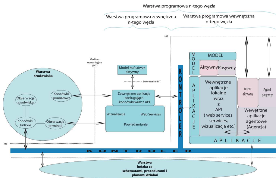
Ryc. 3 Dynamiczne oddziaływanie pomiędzy warstwami z wyszczególnieniem stosu programowego w warstwie programowej n-tego węzła [Opracowanie własne]
